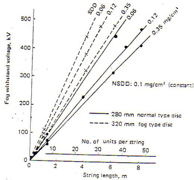
شکل (۳) - رابطه طول زنجیره مقتره ها با ولتاژ ضربه مجاز
