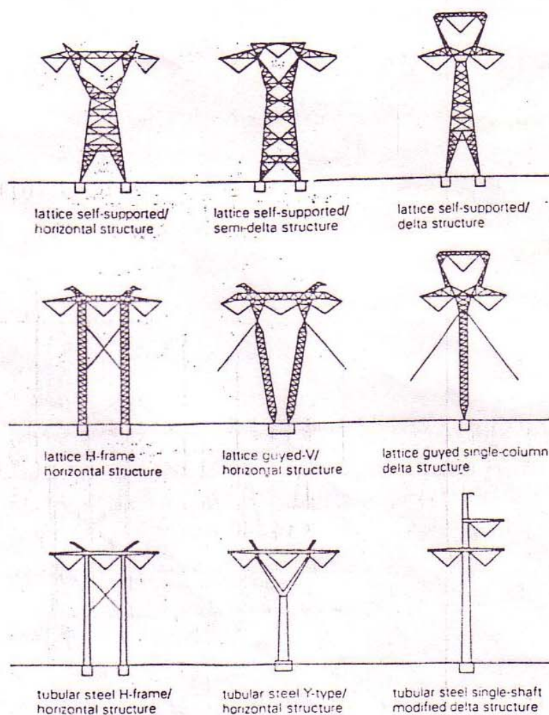
شکل (۴) - چند نمونه از برج‌های کمپاکت و مبهاری (با وضعیت جابجنداری هادی‌ها بصورت مثلثی و افقی)
