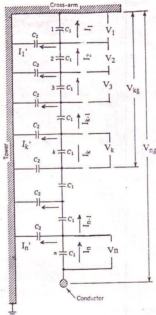
شکل (۱) - مدار معادل زنجیره مقره های خطوط انتقال نیرو در شرایط تمیز بودن مقره ها
