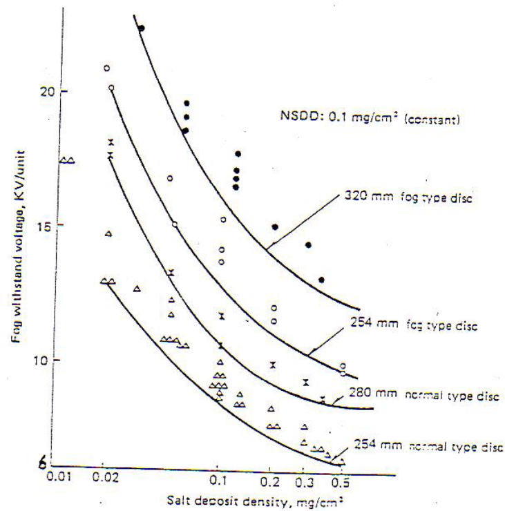
شکل (۴) - رابطه ولتاژ مجاز و میزان املاح برای چند نمونه از مقتره های نوع بشقابی معمولی و ضد مه
