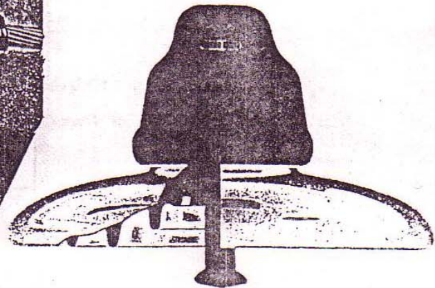
برش عرضی یک نمونه از مقره بشقابی
